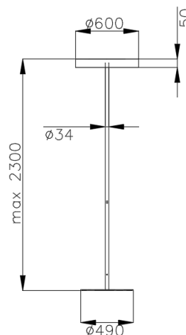
ГАБАРИТНЫЙ ЧЕРТЕЖ
