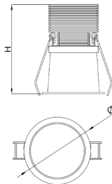
ГАБАРИТНЫЙ ЧЕРТЕЖ
