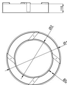
ГАБАРИТНЫЙ ЧЕРТЕЖ
