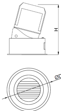
ГАБАРИТНЫЙ ЧЕРТЕЖ
