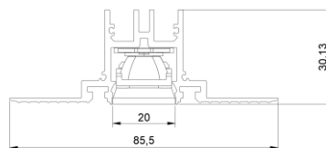
ГАБАРИТНЫЙ ЧЕРТЕЖ
