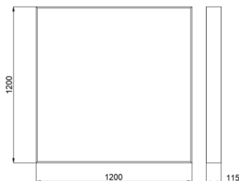
ГАБАРИТНЫЙ ЧЕРТЕЖ
