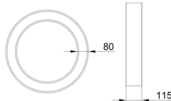
ГАБАРИТНЫЙ ЧЕРТЕЖ
