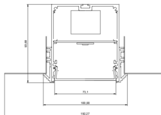
ГАБАРИТНЫЙ ЧЕРТЕЖ
