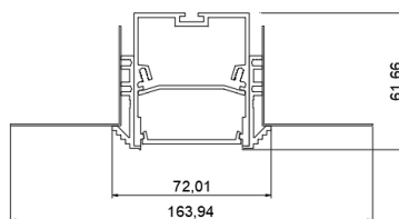
ГАБАРИТНЫЙ ЧЕРТЕЖ
