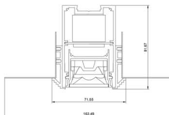
ГАБАРИТНЫЙ ЧЕРТЕЖ
