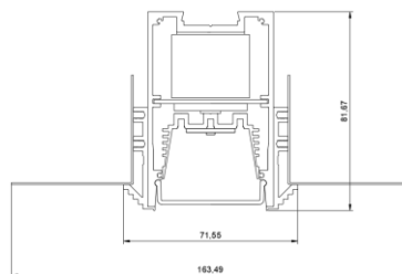
ГАБАРИТНЫЙ ЧЕРТЕЖ
