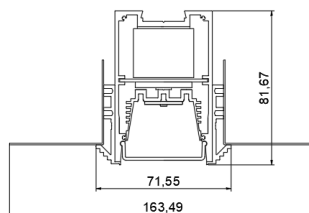
ГАБАРИТНЫЙ ЧЕРТЕЖ
