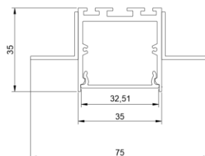
ГАБАРИТНЫЙ ЧЕРТЕЖ
