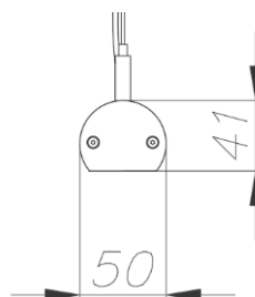
ГАБАРИТНЫЙ ЧЕРТЕЖ
