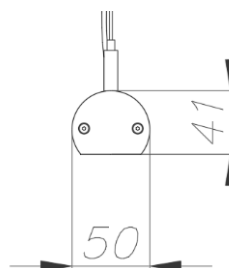
ГАБАРИТНЫЙ ЧЕРТЕЖ
