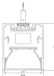
ГАБАРИТНЫЙ ЧЕРТЕЖ
