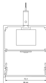
ГАБАРИТНЫЙ ЧЕРТЕЖ
