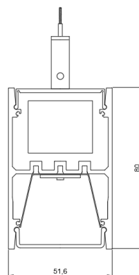
ГАБАРИТНЫЙ ЧЕРТЕЖ
