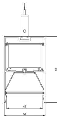
ГАБАРИТНЫЙ ЧЕРТЕЖ
