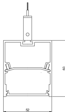
ГАБАРИТНЫЙ ЧЕРТЕЖ
