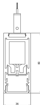
ГАБАРИТНЫЙ ЧЕРТЕЖ
