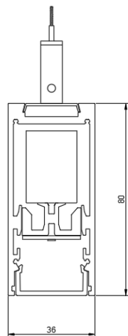
ГАБАРИТНЫЙ ЧЕРТЕЖ
