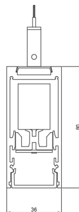
ГАБАРИТНЫЙ ЧЕРТЕЖ
