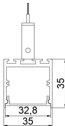
ГАБАРИТНЫЙ ЧЕРТЕЖ
