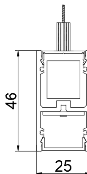
ГАБАРИТНЫЙ ЧЕРТЕЖ
