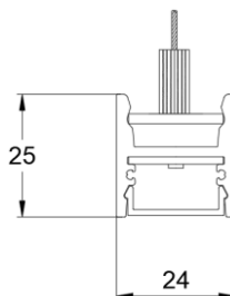
ГАБАРИТНЫЙ ЧЕРТЕЖ
