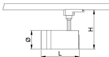
ГАБАРИТНЫЙ ЧЕРТЕЖ
