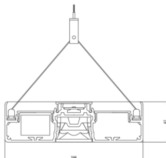
ГАБАРИТНЫЙ ЧЕРТЕЖ
