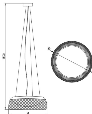
ГАБАРИТНЫЙ ЧЕРТЕЖ
