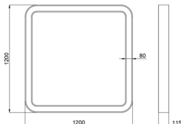
ГАБАРИТНЫЙ ЧЕРТЕЖ
