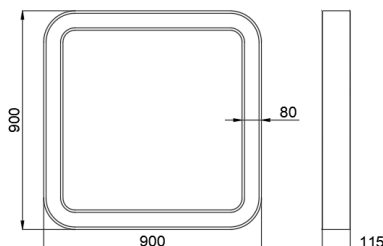
ГАБАРИТНЫЙ ЧЕРТЕЖ
