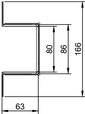
Сечение
