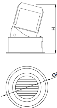
ГАБАРИТНЫЙ ЧЕРТЕЖ
