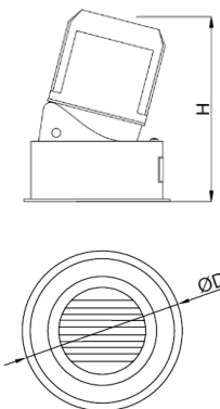
ГАБАРИТНЫЙ ЧЕРТЕЖ
