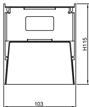
Габаритный чертеж
