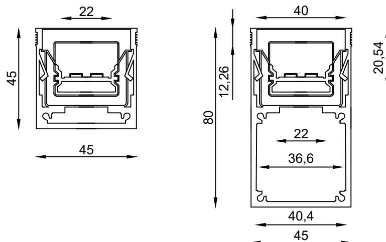
Габаритный чертеж
