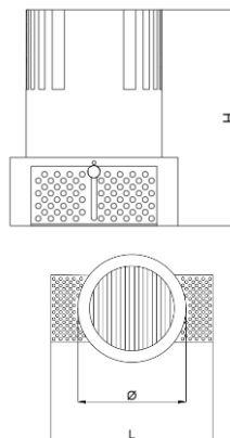
ГАБАРИТНЫЙ ЧЕРТЕЖ
