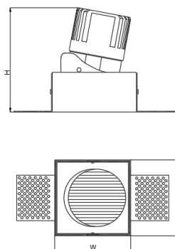
ГАБАРИТНЫЙ ЧЕРТЕЖ
