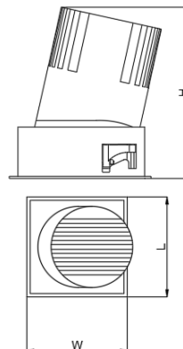
ГАБАРИТНЫЙ ЧЕРТЕЖ
