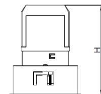
ГАБАРИТНЫЙ ЧЕРТЕЖ
