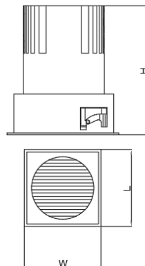
ГАБАРИТНЫЙ ЧЕРТЕЖ
