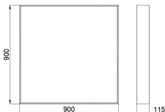
ГАБАРИТНЫЙ ЧЕРТЕЖ
