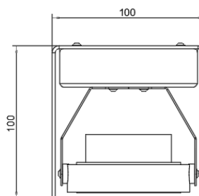
ГАБАРИТНЫЙ ЧЕРТЕЖ
