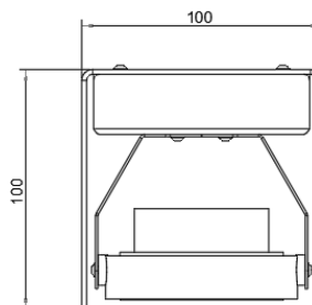
ГАБАРИТНЫЙ ЧЕРТЕЖ
