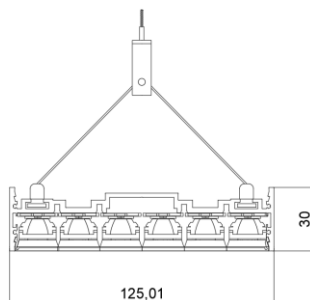
ГАБАРИТНЫЙ ЧЕРТЕЖ
