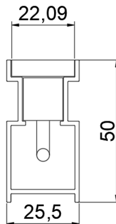
ГАБАРИТНЫЙ ЧЕРТЕЖ
