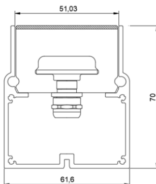
ГАБАРИТНЫЙ ЧЕРТЕЖ
