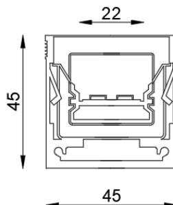
ГАБАРИТНЫЙ ЧЕРТЕЖ
