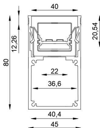
ГАБАРИТНЫЙ ЧЕРТЕЖ
