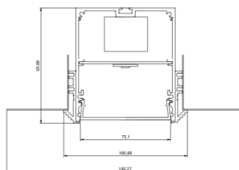
ГАБАРИТНЫЙ ЧЕРТЕЖ
