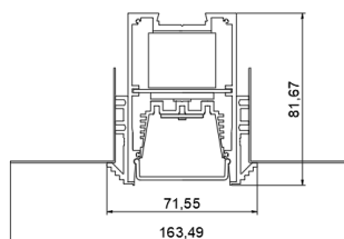
ГАБАРИТНЫЙ ЧЕРТЕЖ
